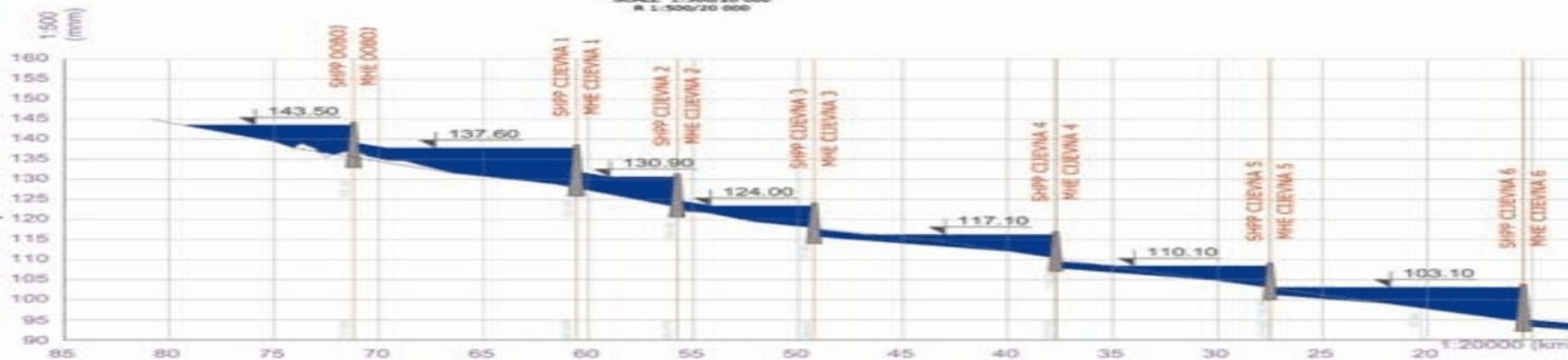
LONGITUDINAL SECTION PODUŽNI PROFIL SCALE 1 : 300/20 000 R 1 : 300/20 000
